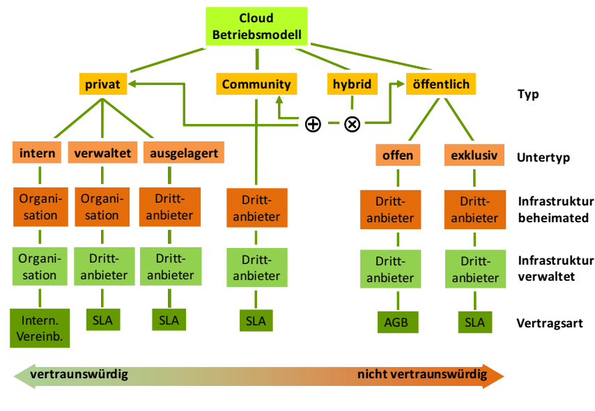
Abbildung I.1.2 Taxonomie der Cloud-Betriebsmodelle.
